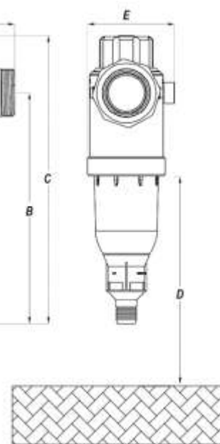
PuliFIL ühendused 1"1/2 - 2"
