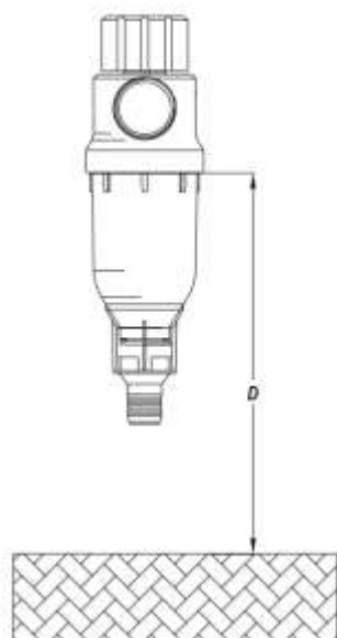
PuliFIL ühendus 3/4" - 1" -
